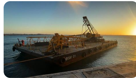
Balsa atracando no TMUT para instalação do guindaste
