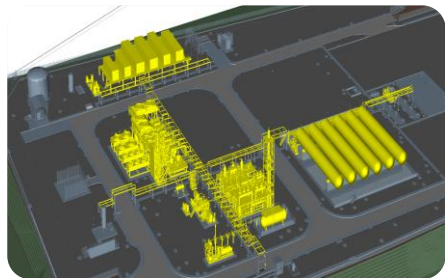
Layout da Planta
