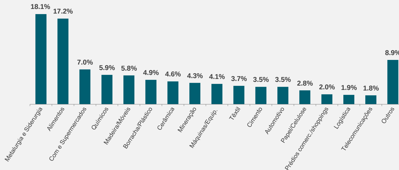
Volume contratado para clientes livres em 2024: 2.014 MWh
