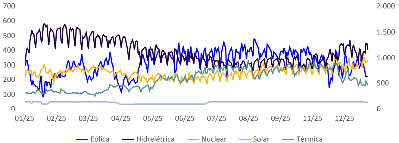
Gráfico 7 - Energia gerada SIN – Sistema Interligado Nacional (GWh)
